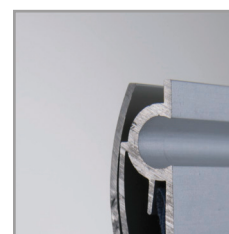
Aufhängung mit Aluklemmschiene
